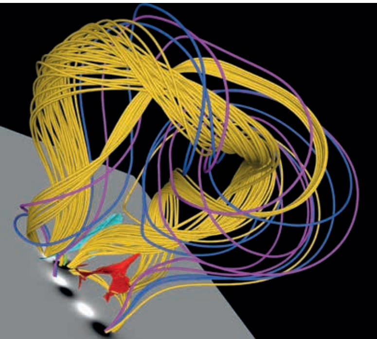
Mit Computernmodellen stellen Forscher Sonneneruptionen nach und berechnen die wirkenden physikalischen Kräfte.
