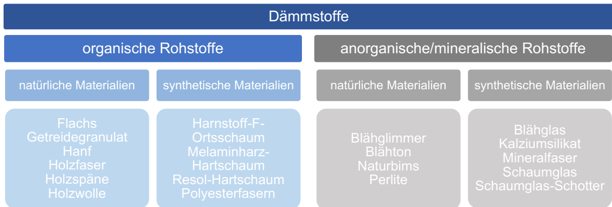
Abbildung 3: Kategorisierung von Dämmstoffen (Danner, 2010, S. 10, eigene Darstellung).
